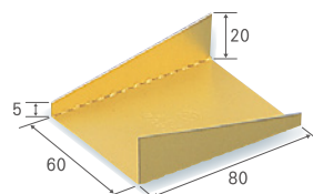
メタル 60×80
