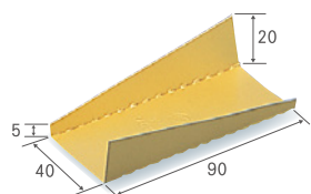
メタル 40×90
