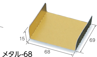
メタル-68
